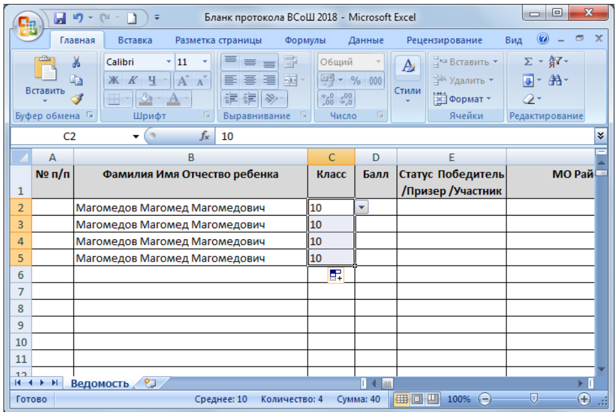
Рисунок 2. Автозаполнение.
